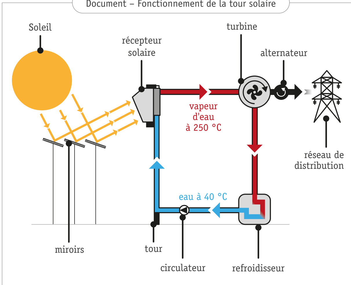
Document – Fonctionnement de la tour solaire
