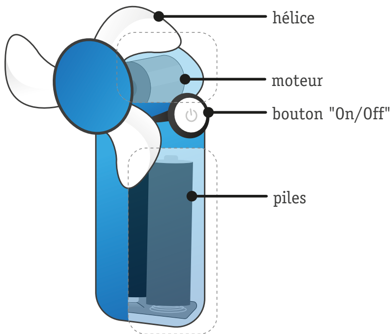
Document – Schéma simplifié du ventilateur de Dorothée
